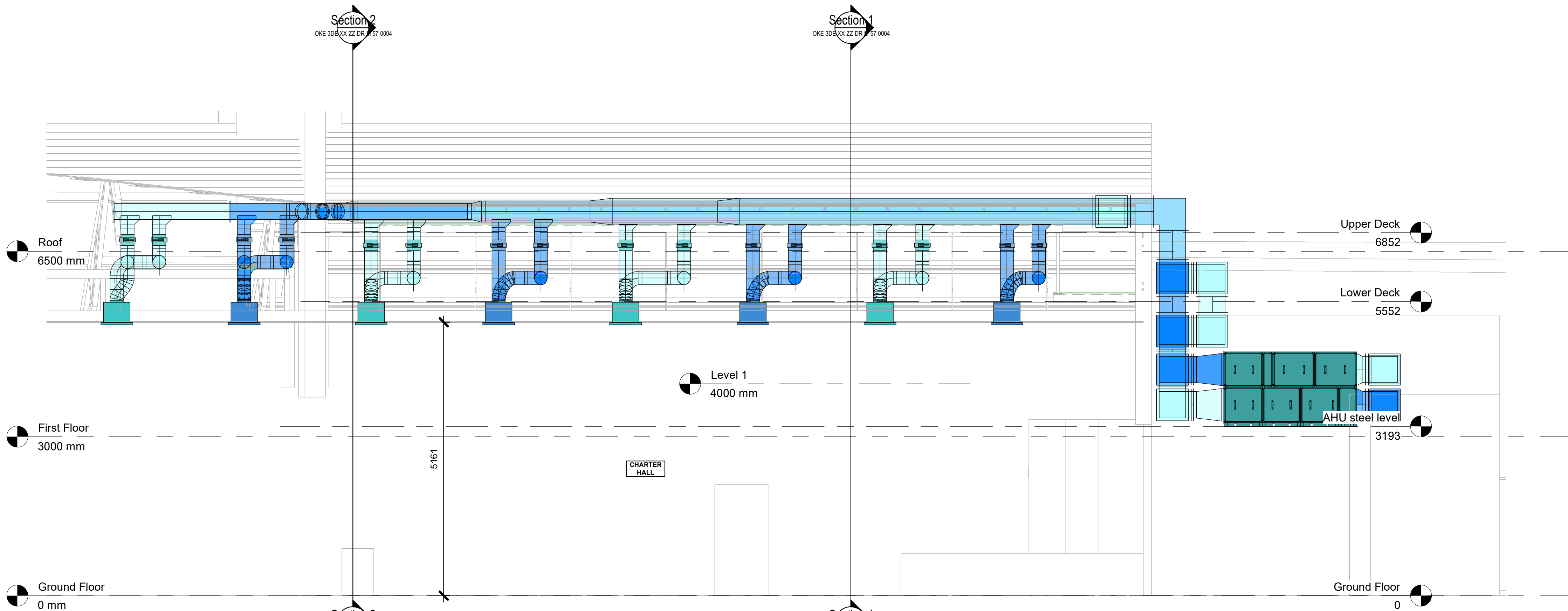
3 Section 3 1 : 50
