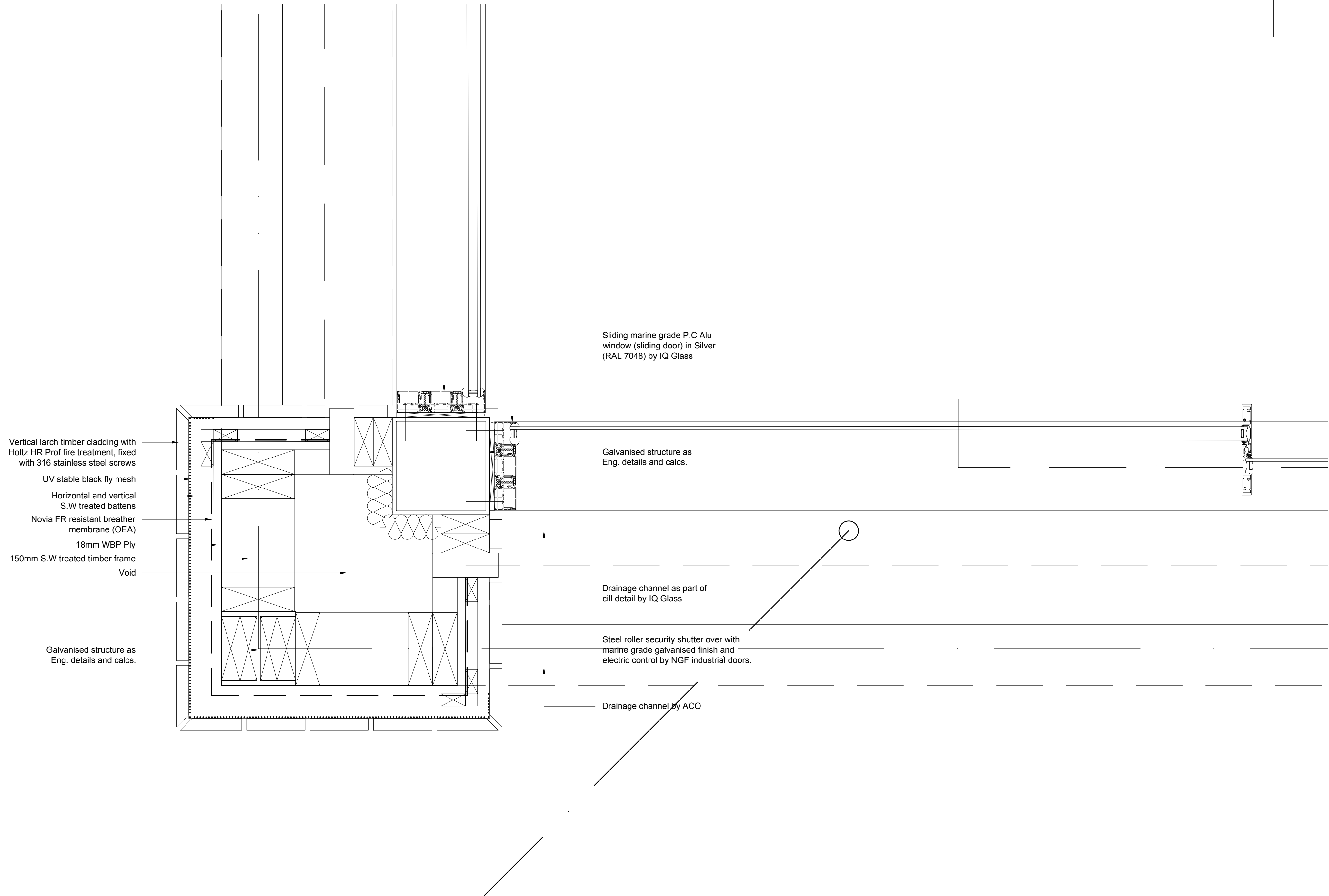
Sliding door detail 1:5
