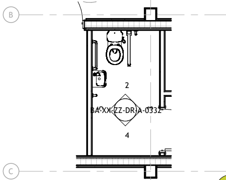
1 F06 - Dis WC Scale 1 : 50
