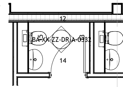
11 F08 - WC Scale 1 : 50
