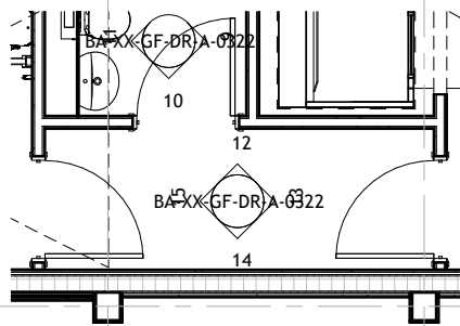
3 G08 - WC Lobby Scale 1 : 50
