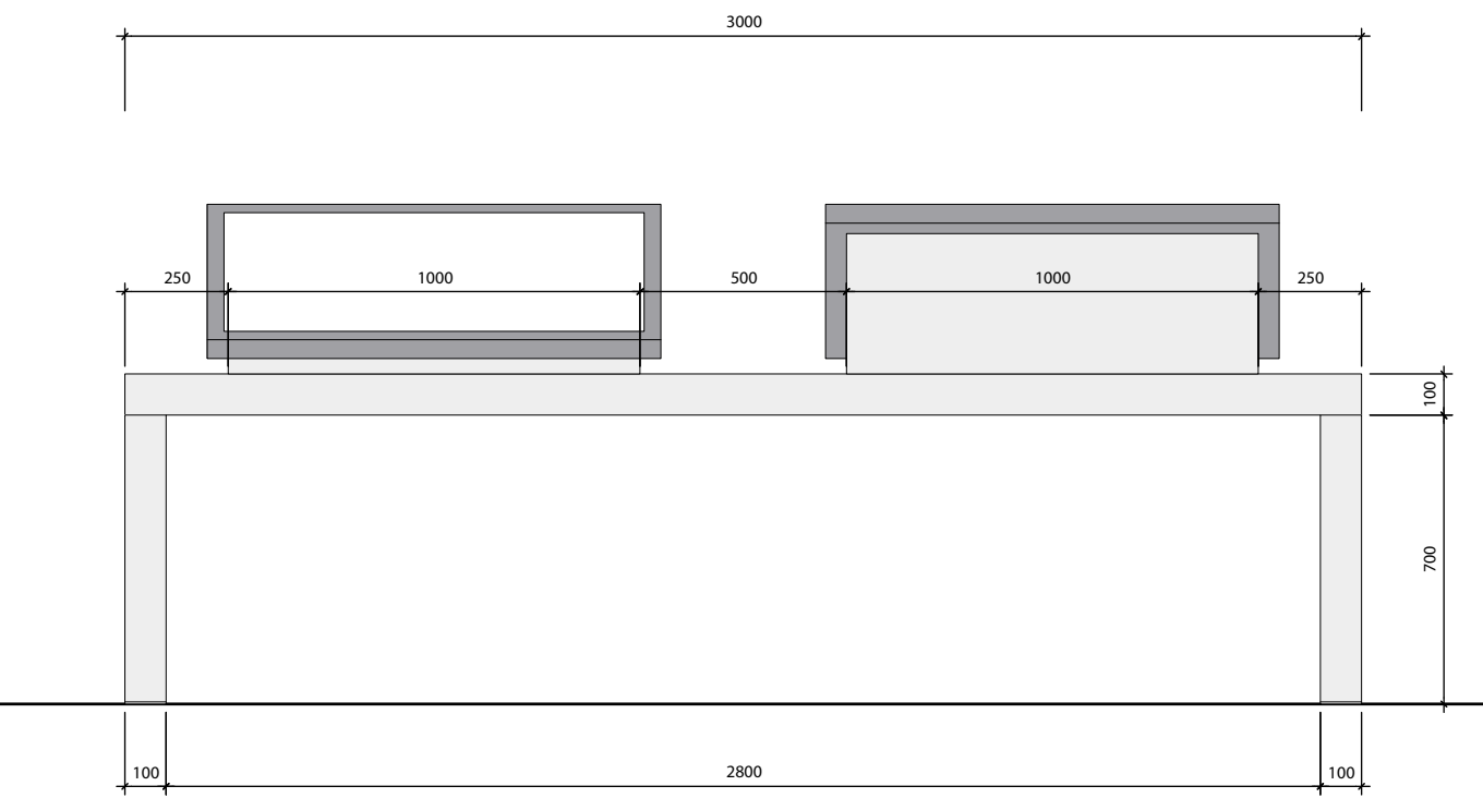
02 SB07 Table Elevation
