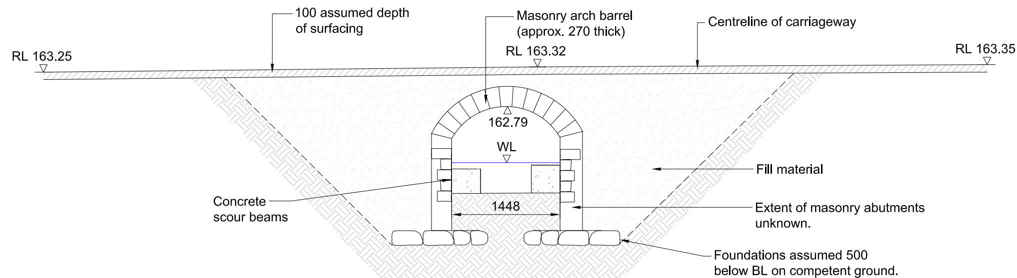
Section A-A 1:50
