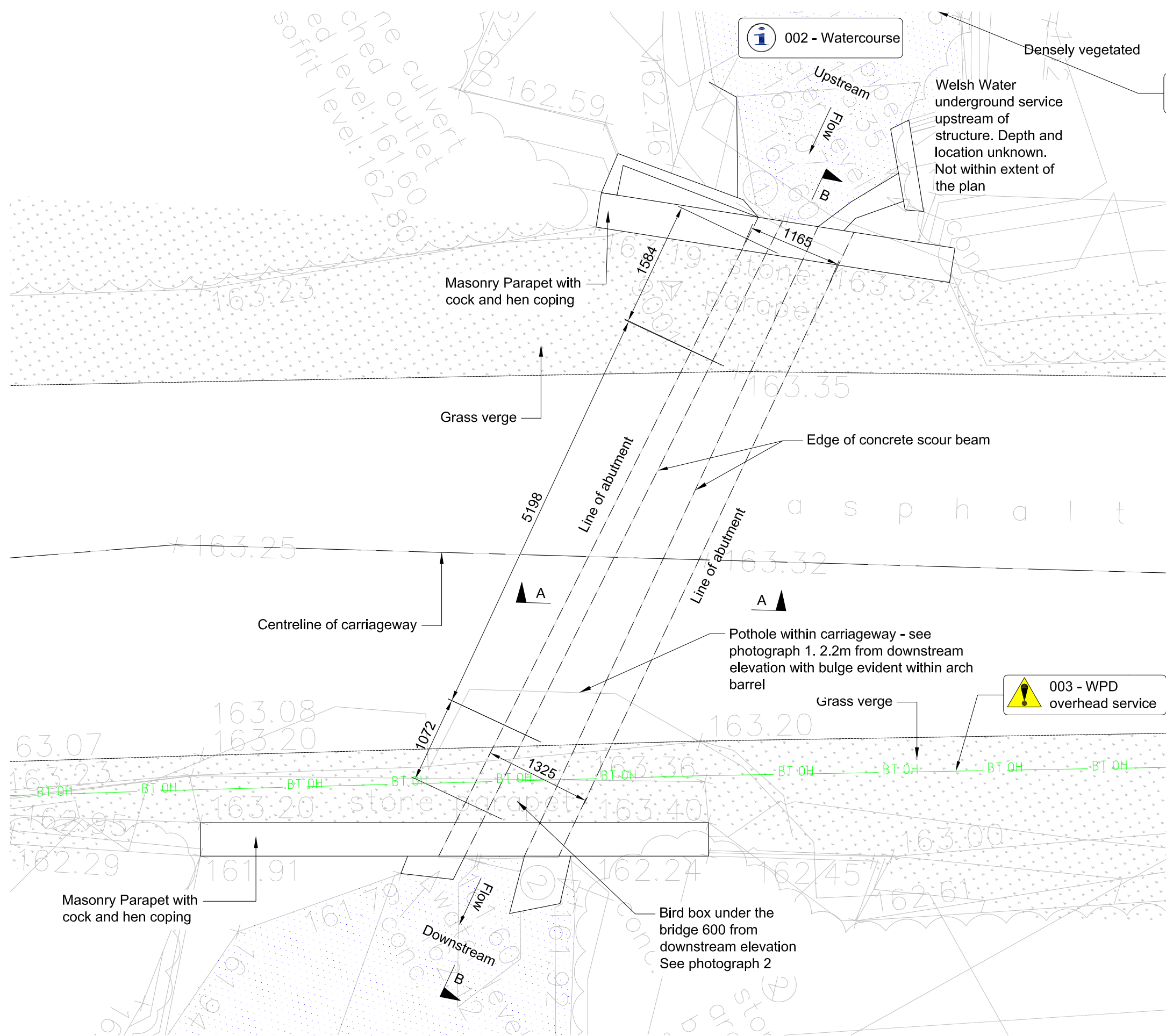
Plan 1:50
