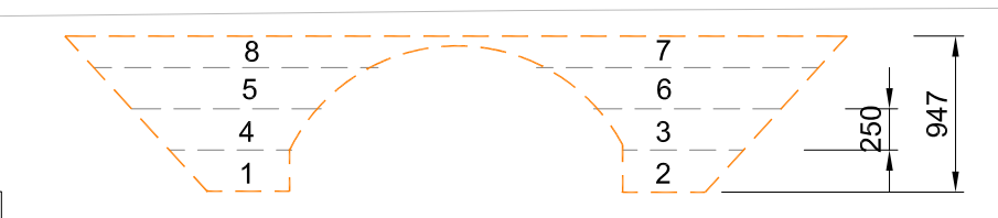
Sequence of concrete Pour (Balanced Pour) 1:50
