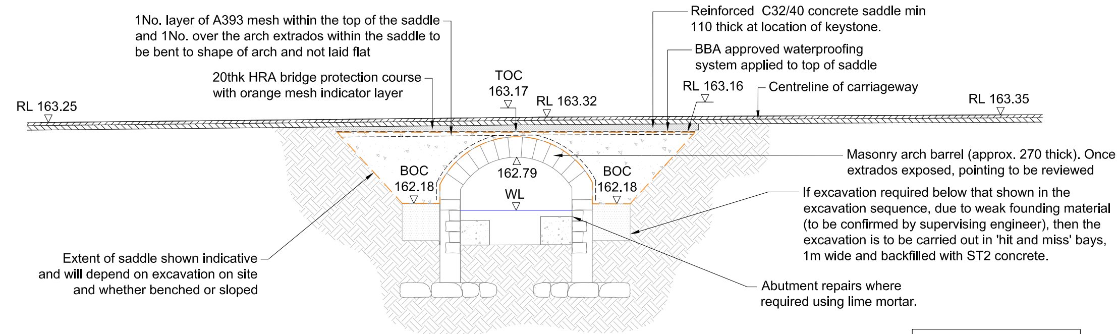
Section A-A 1:50
