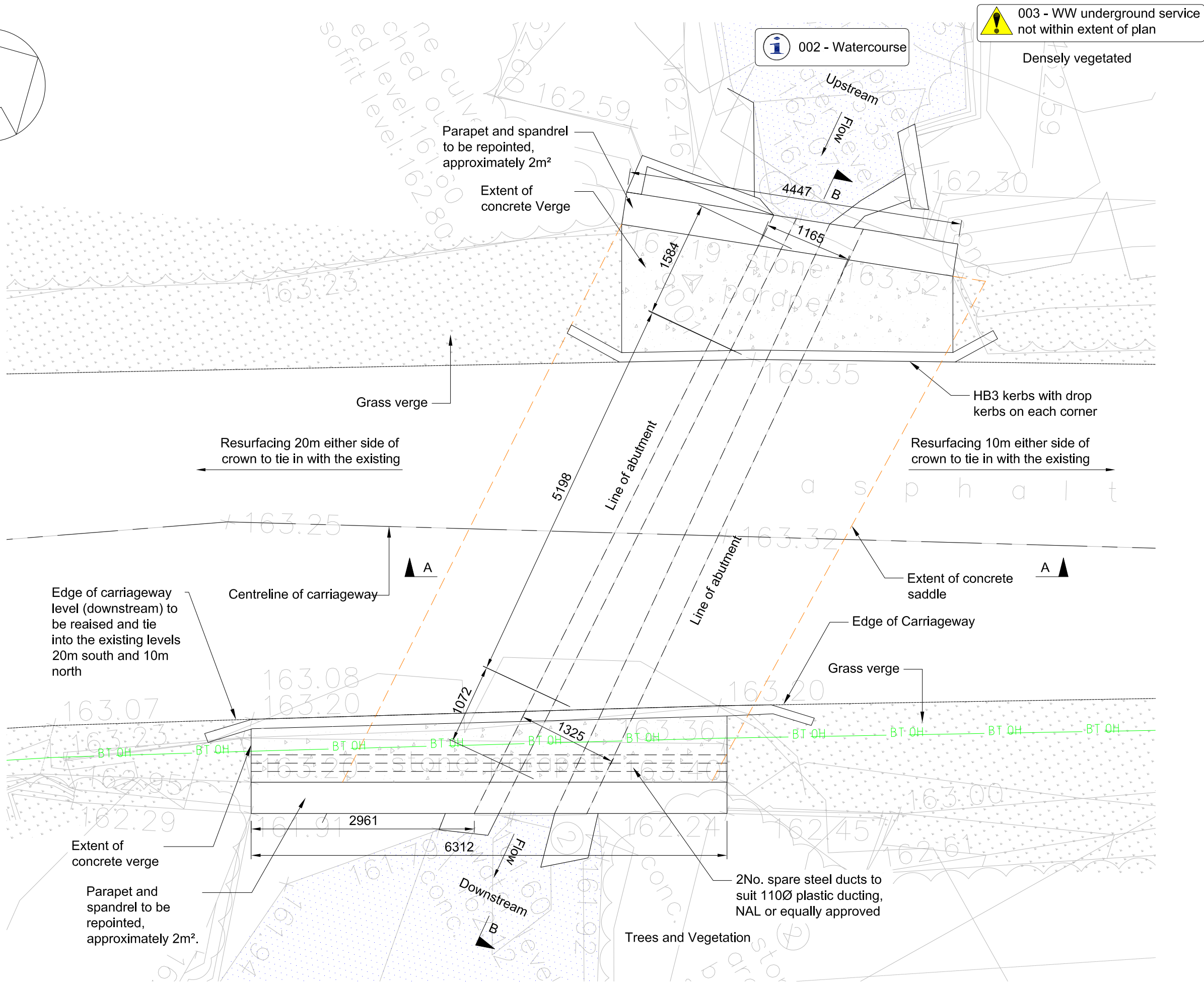
Plan 1:50
