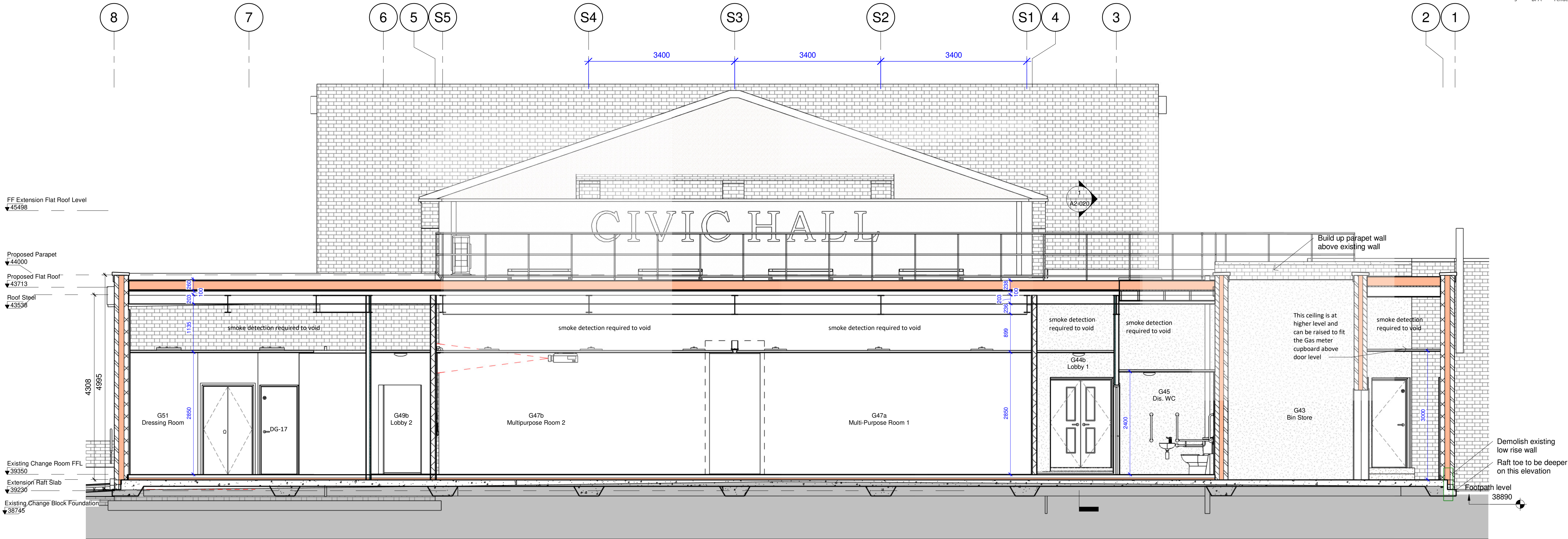
Section A-A 1 : 50
