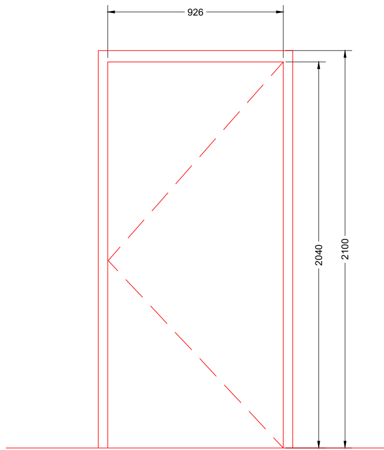
Door Type E Door D13 (ambulant toilet cubicle)
