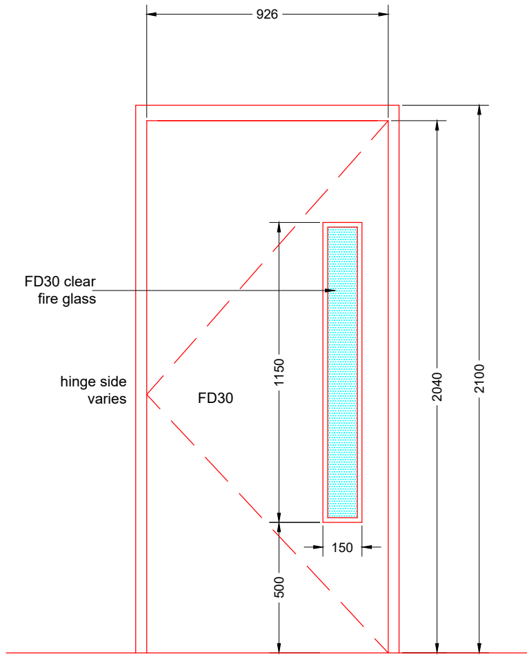
Door Type A Doors D1, D3, D4, D5, D9, D10 & D25
