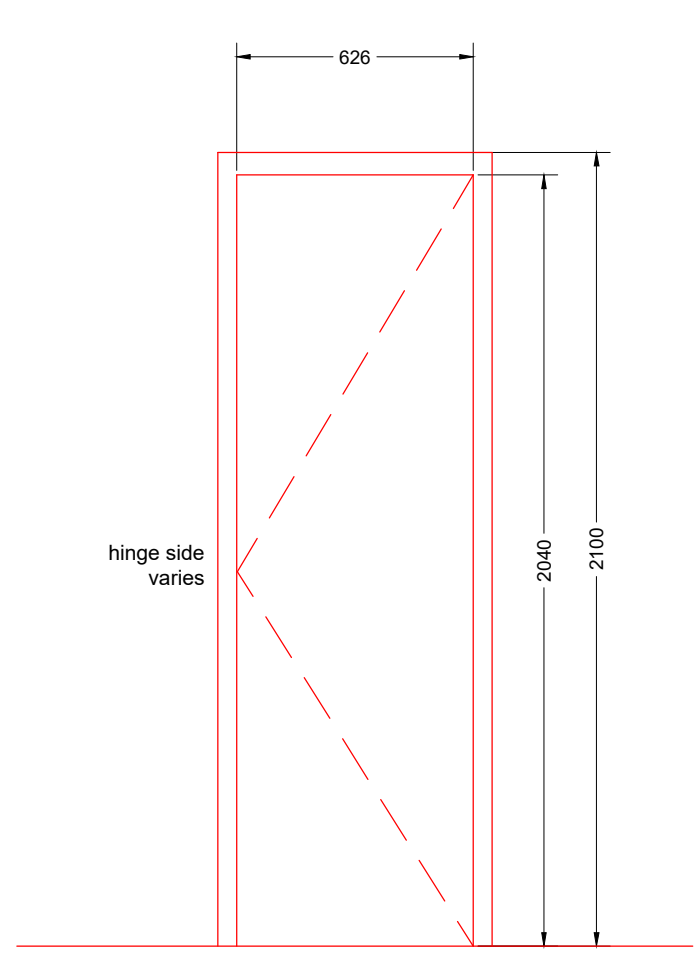
Door Type D Doors D11, D12, D14 & D15 (toilet cubicles)
