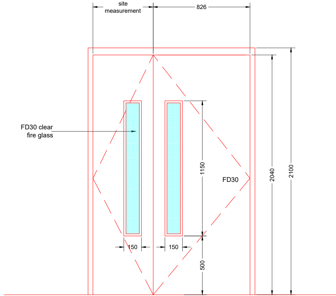
Door Type D Doors D11, D12, D14 & D15 (toilet cubicles)
