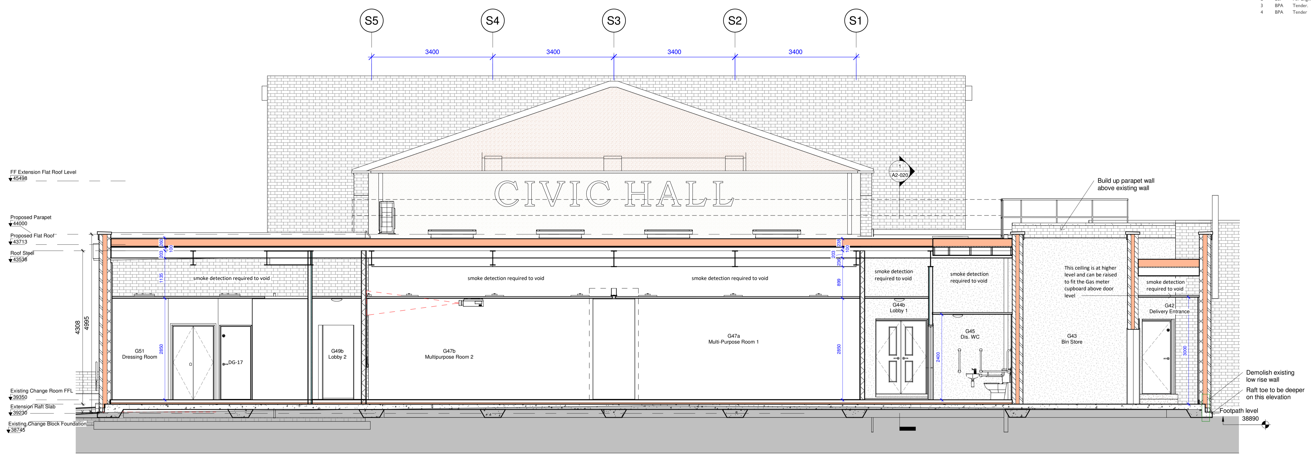
Section A-A 1 : 50
