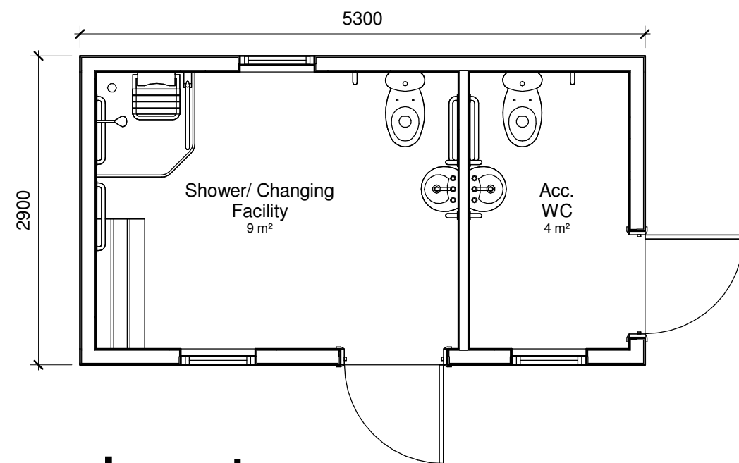
1 Layout 1 : 50
