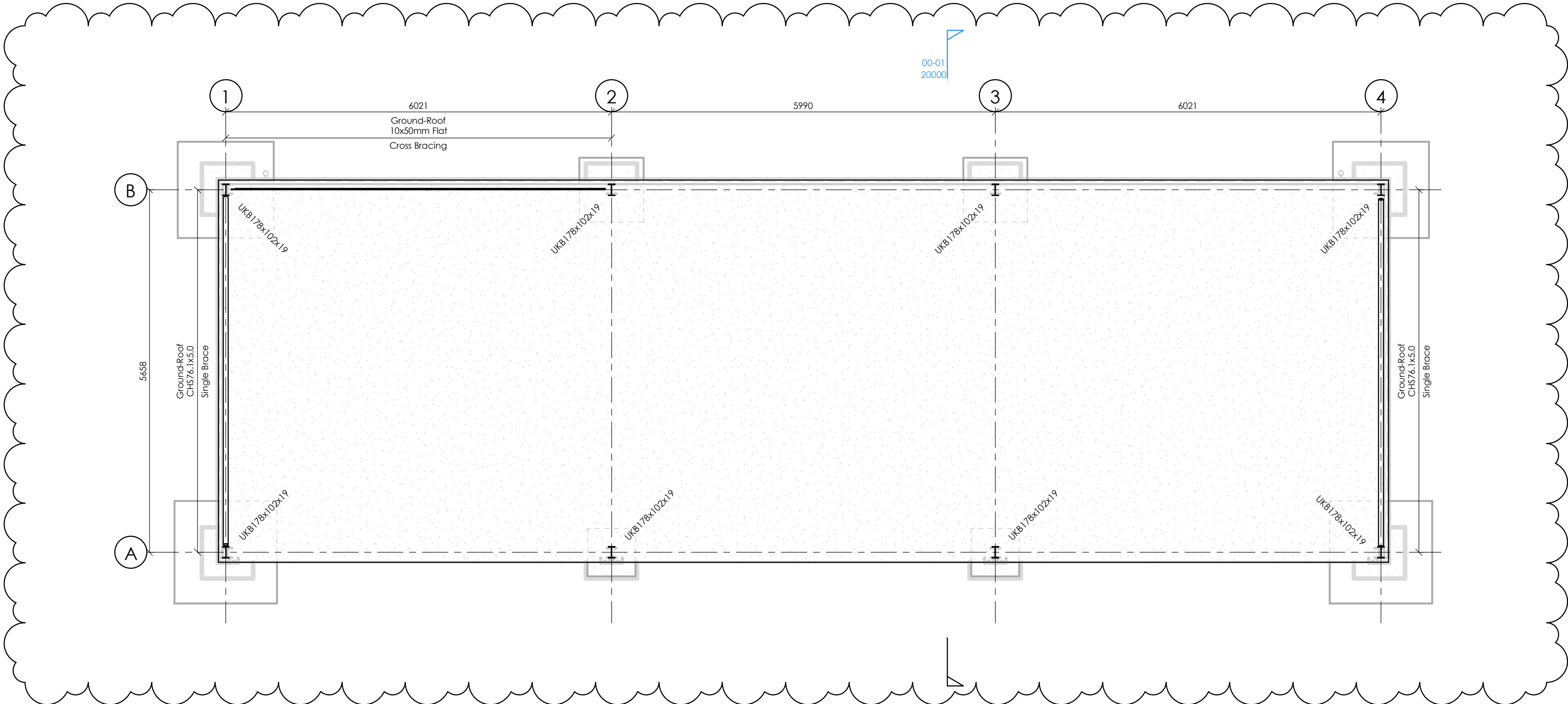
COLUMN LAYOUT 1 : 50
