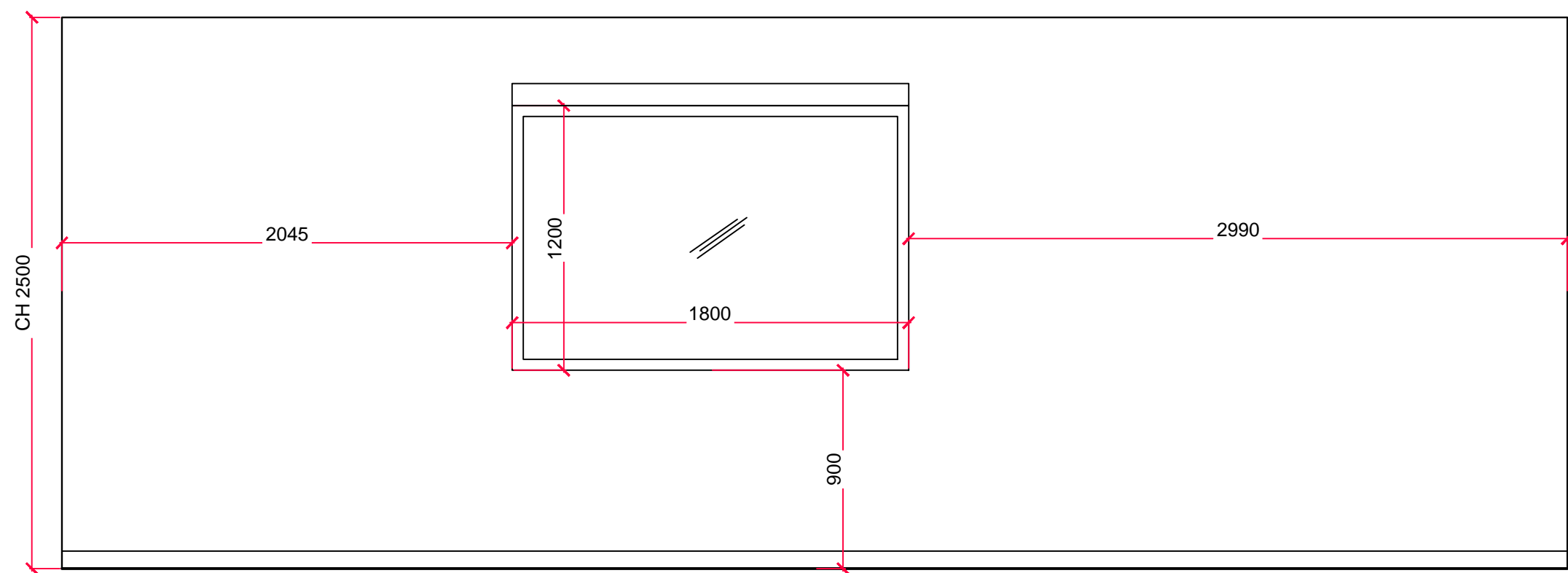
3 ELEVATION - C C Scale: 1:25 @ A1 1:50 @ A3
