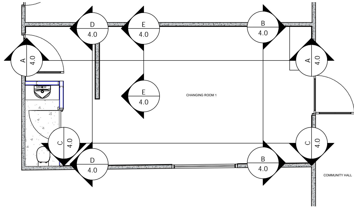
1 KEY - ELEVATION PLAN Scale: 1:50 @ A1 1:100 @ A3
