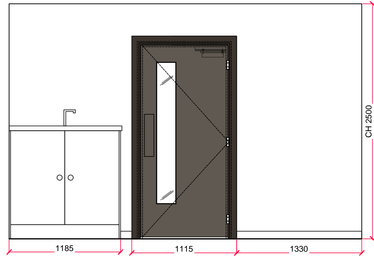
3 ELEVATION - B B Scale: 1:25 @ A1 1:50 @ A3
