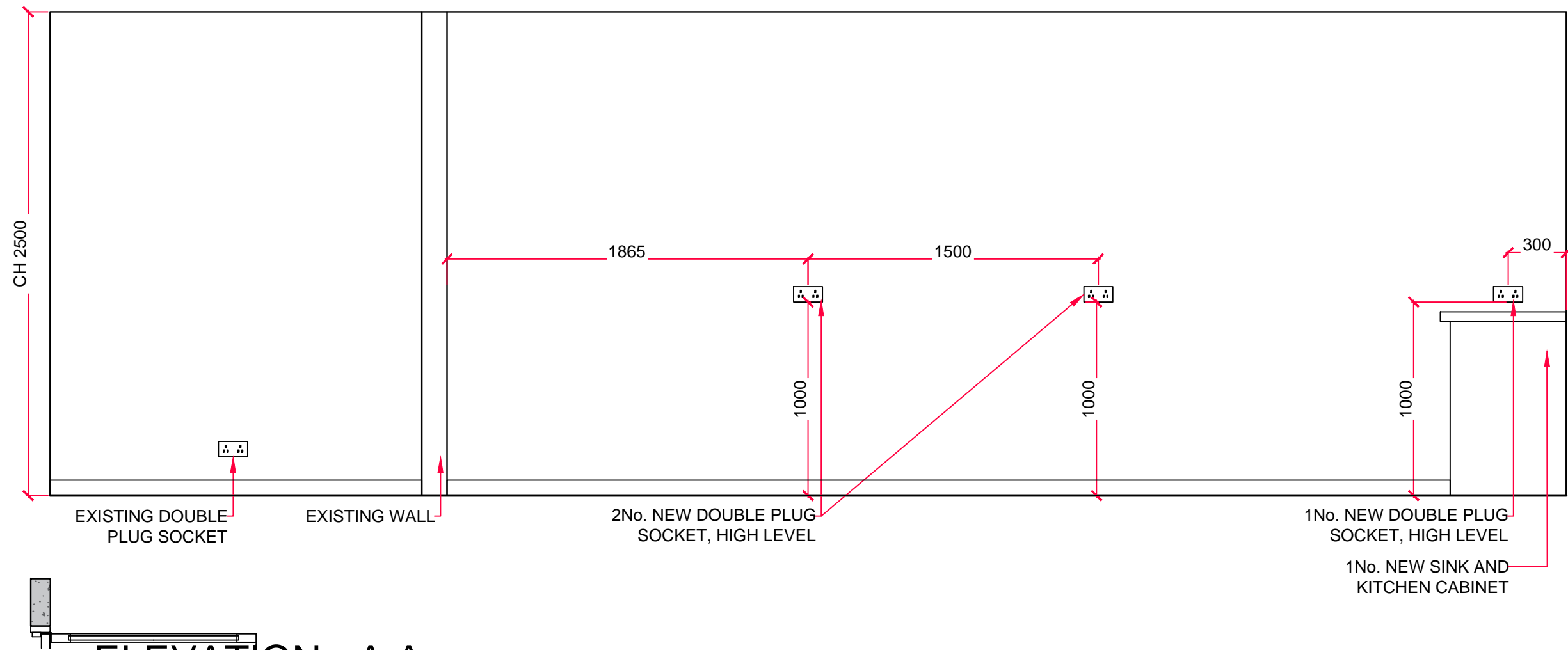
3 ELEVATION - A A Scale: 1:25 @ A1 1:50 @ A3
