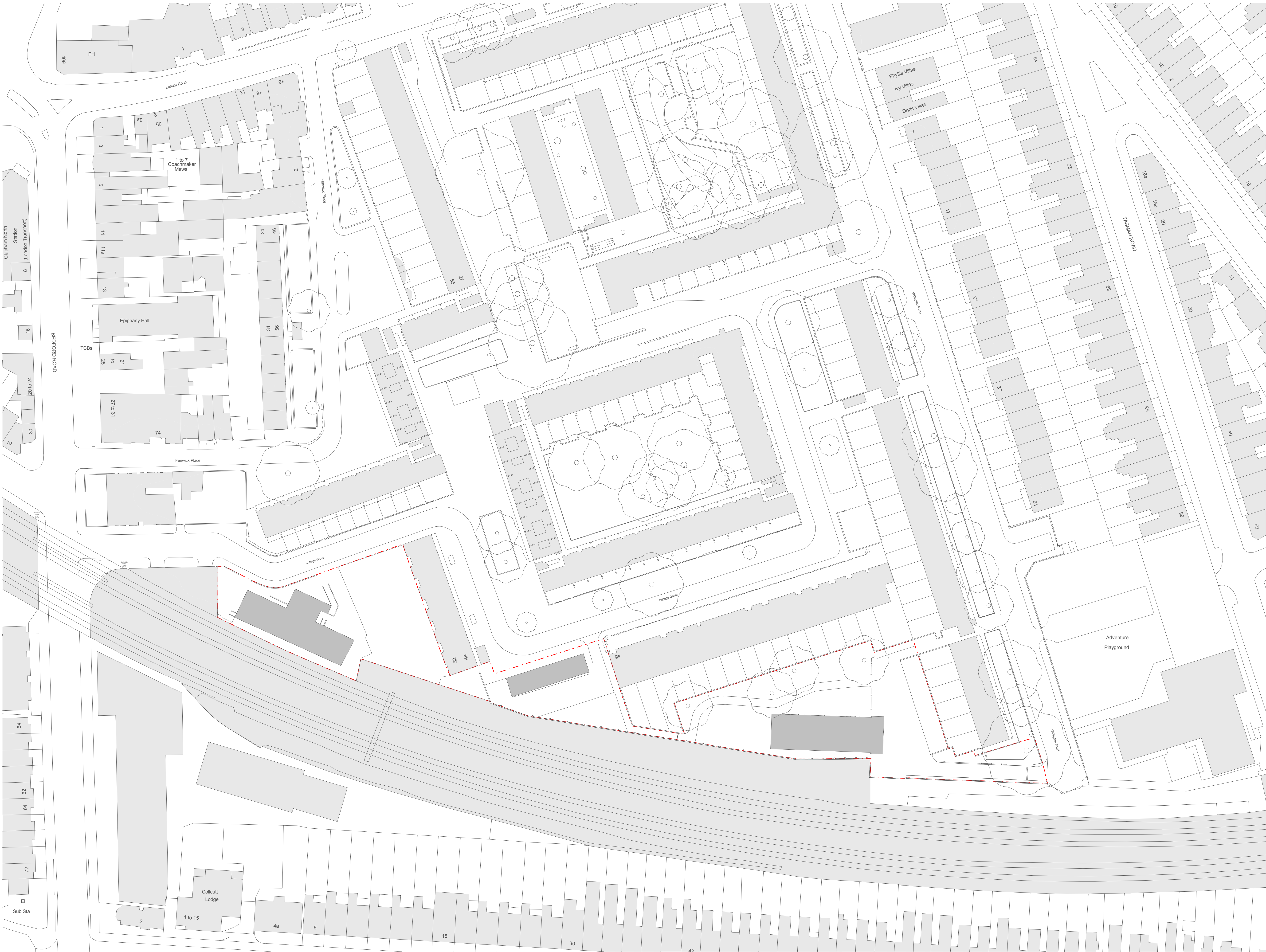
D-1 Existing Site Plan 000-01 1: 500
