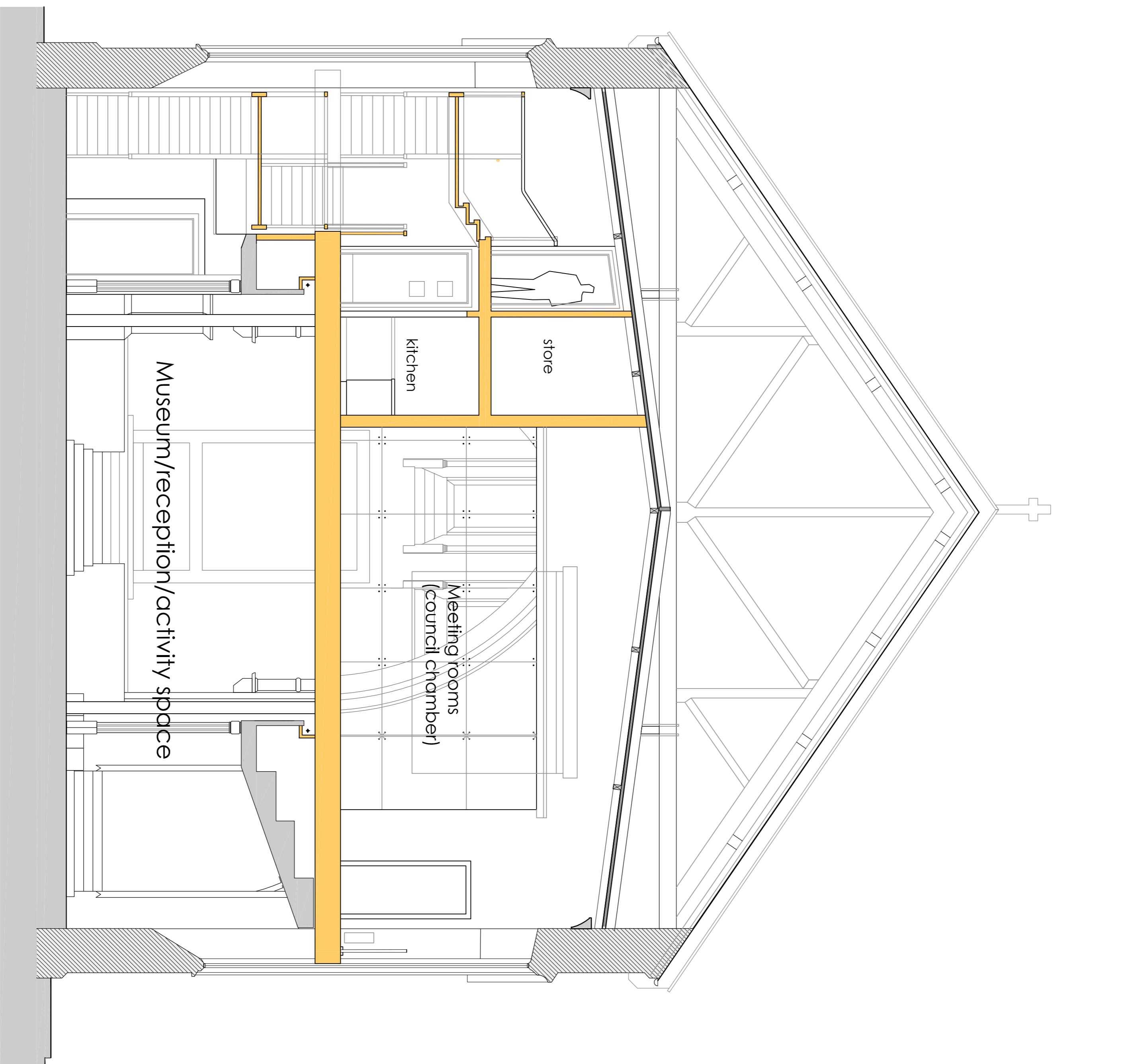
Section D-D
