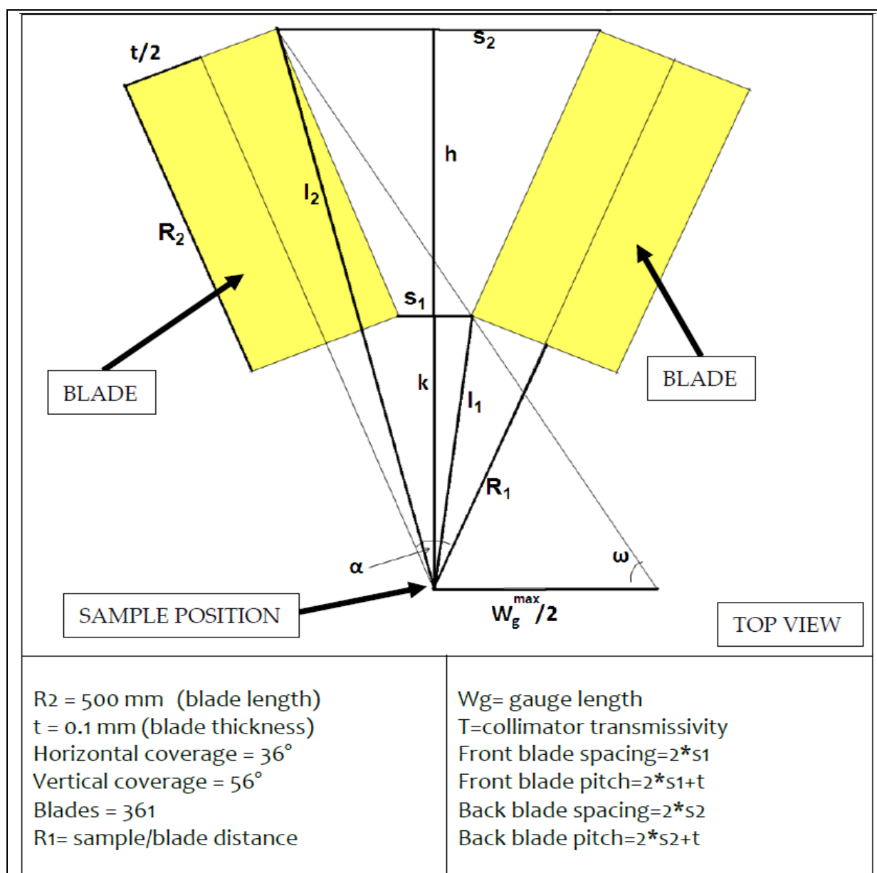
Figure 5 – Blade parameters
