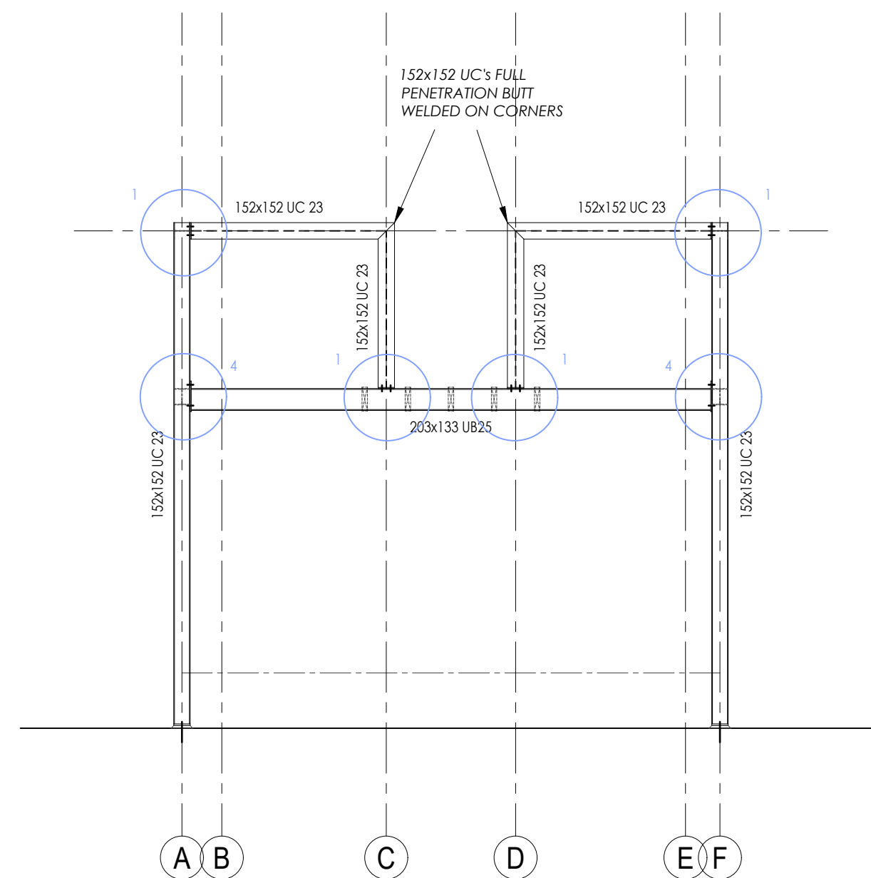
ELEVATION GL 5
