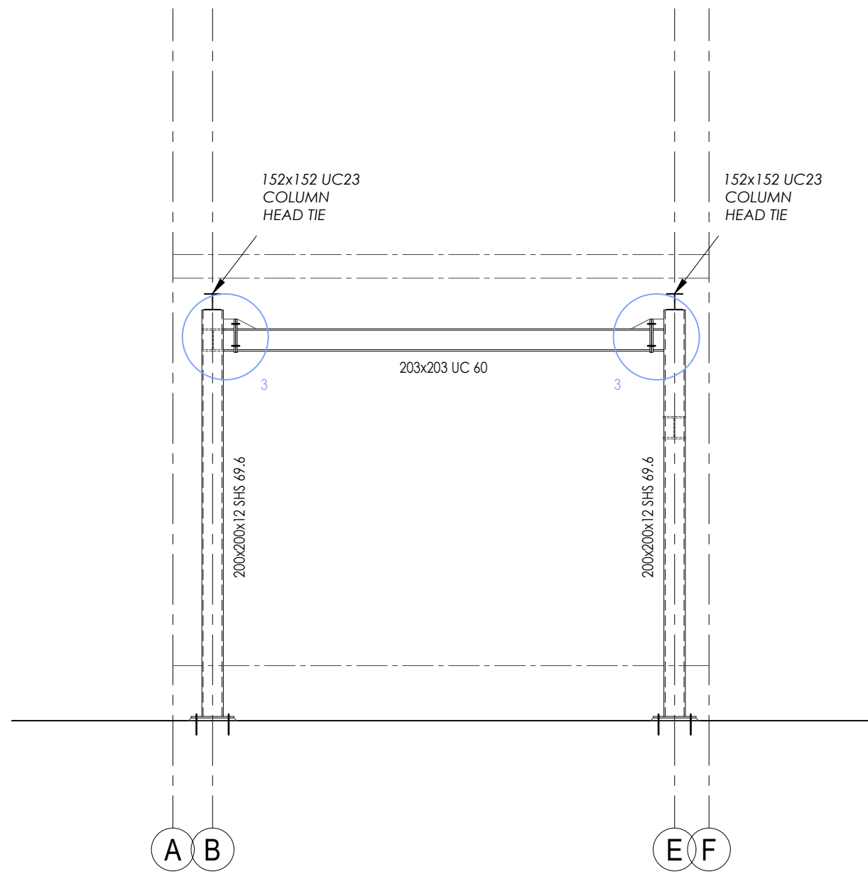
ELEVATION GL 2
