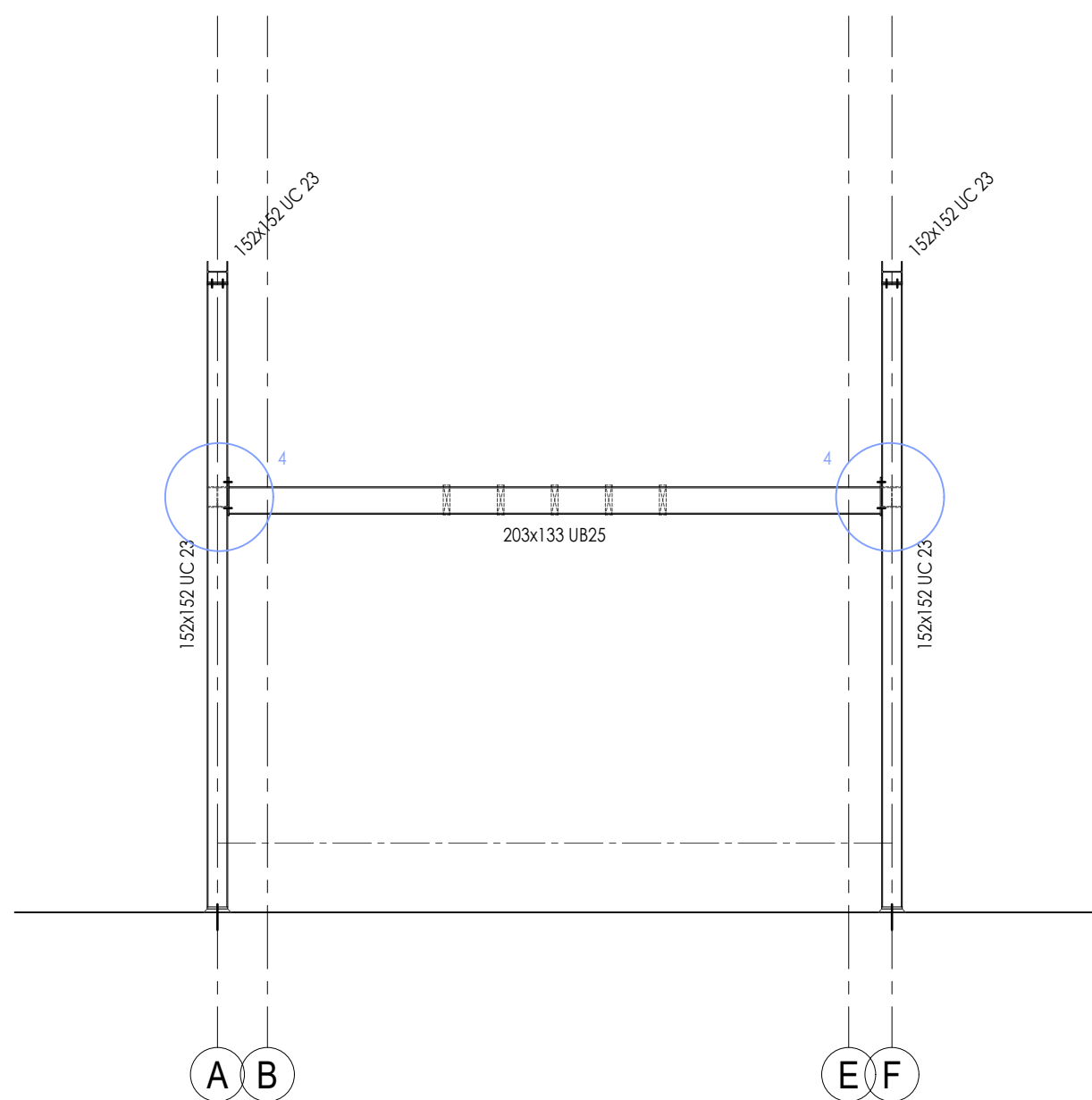
ELEVATION GL 4
