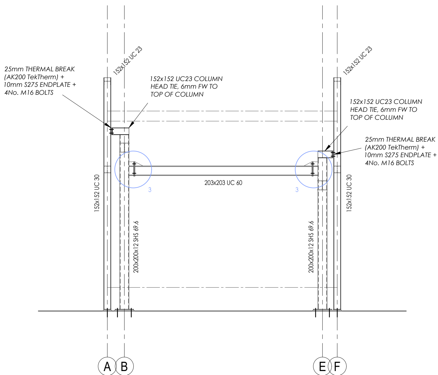
ELEVATION GL 3
