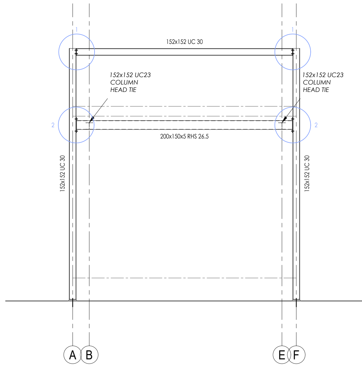
ELEVATION GL 1
