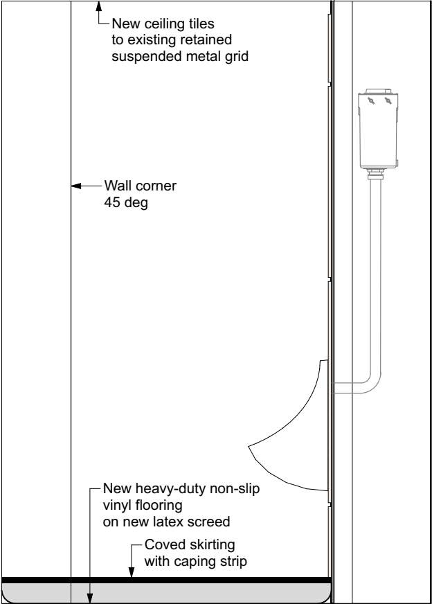
IE-02 07 Men WC 1:20
