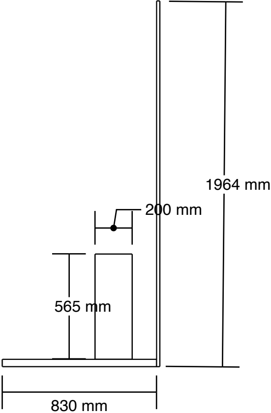
Elevation 2 1:20 @ A3
