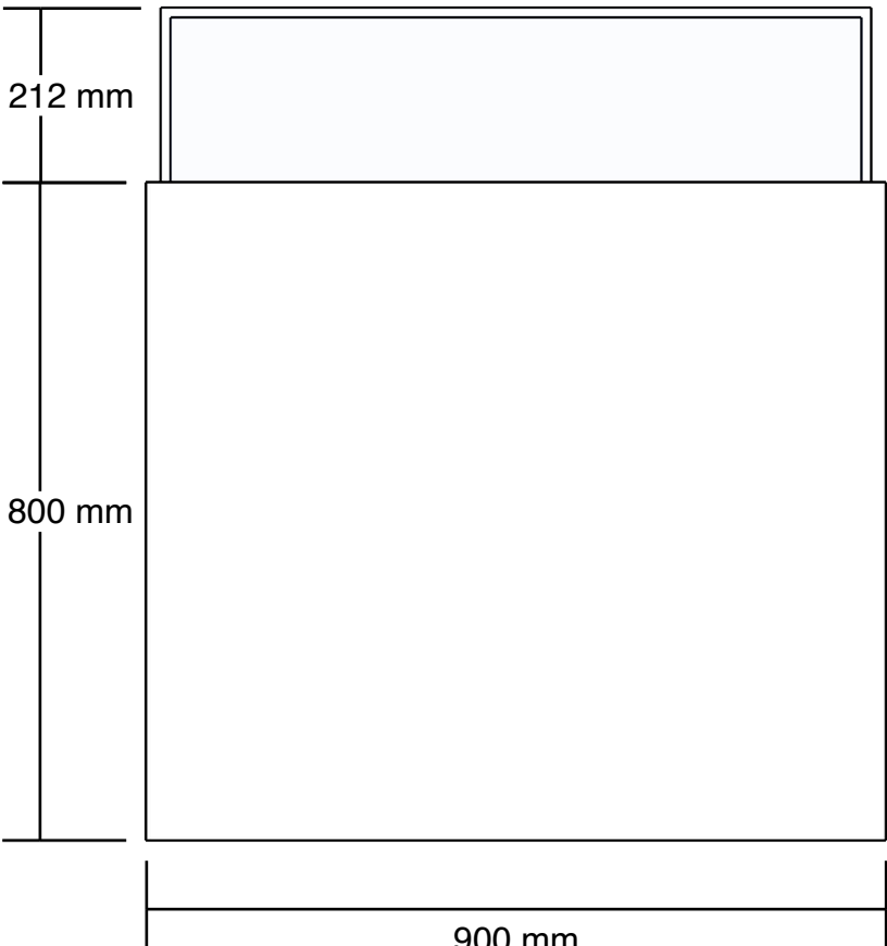
Elevation 2 1:10 @ A3
