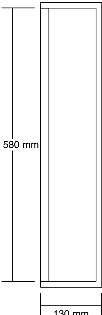
Elevation 2 1:5 @ A3
