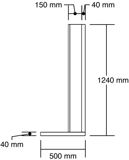
Elevation 2 1:20 @ A3
