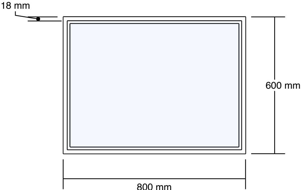
Elevation 1 1:10 @ A3
