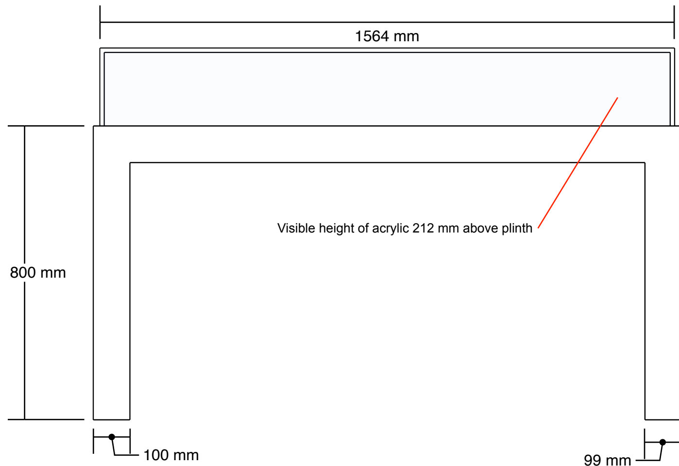
Elevation 1 1:10 @ A3
