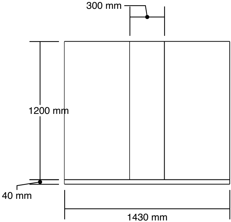
Elevation 1 1:20 @ A3
