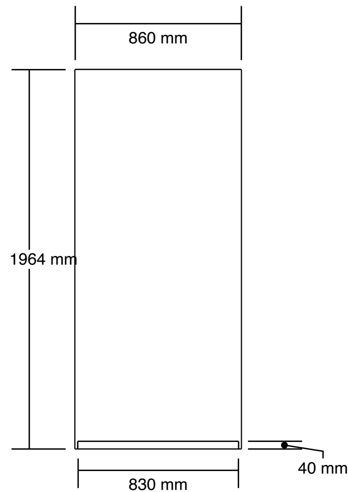
Elevation 1 1:20 @ A3
