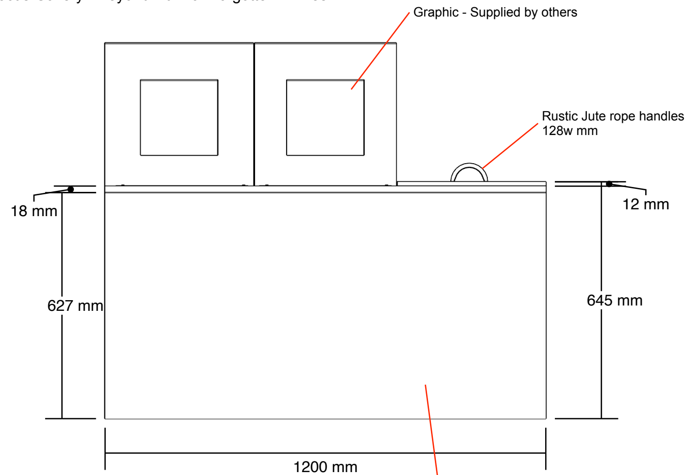
Elevation 1 1:10 @ A3
