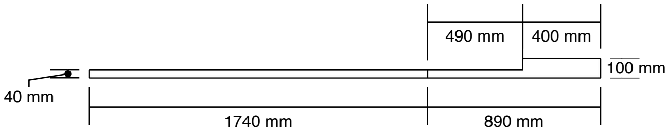
Elevation 1 1:20 @ A3
