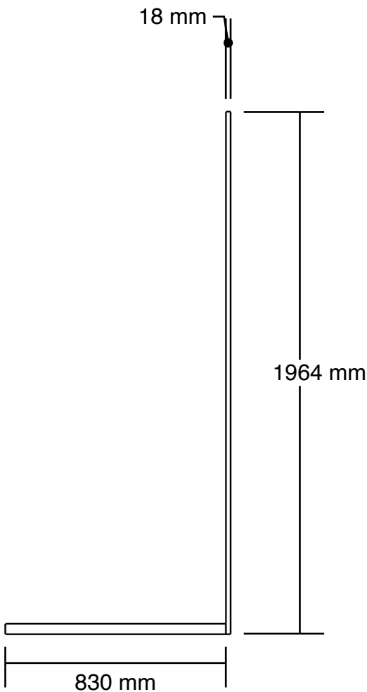
Elevation 2 1:20 @ A3
