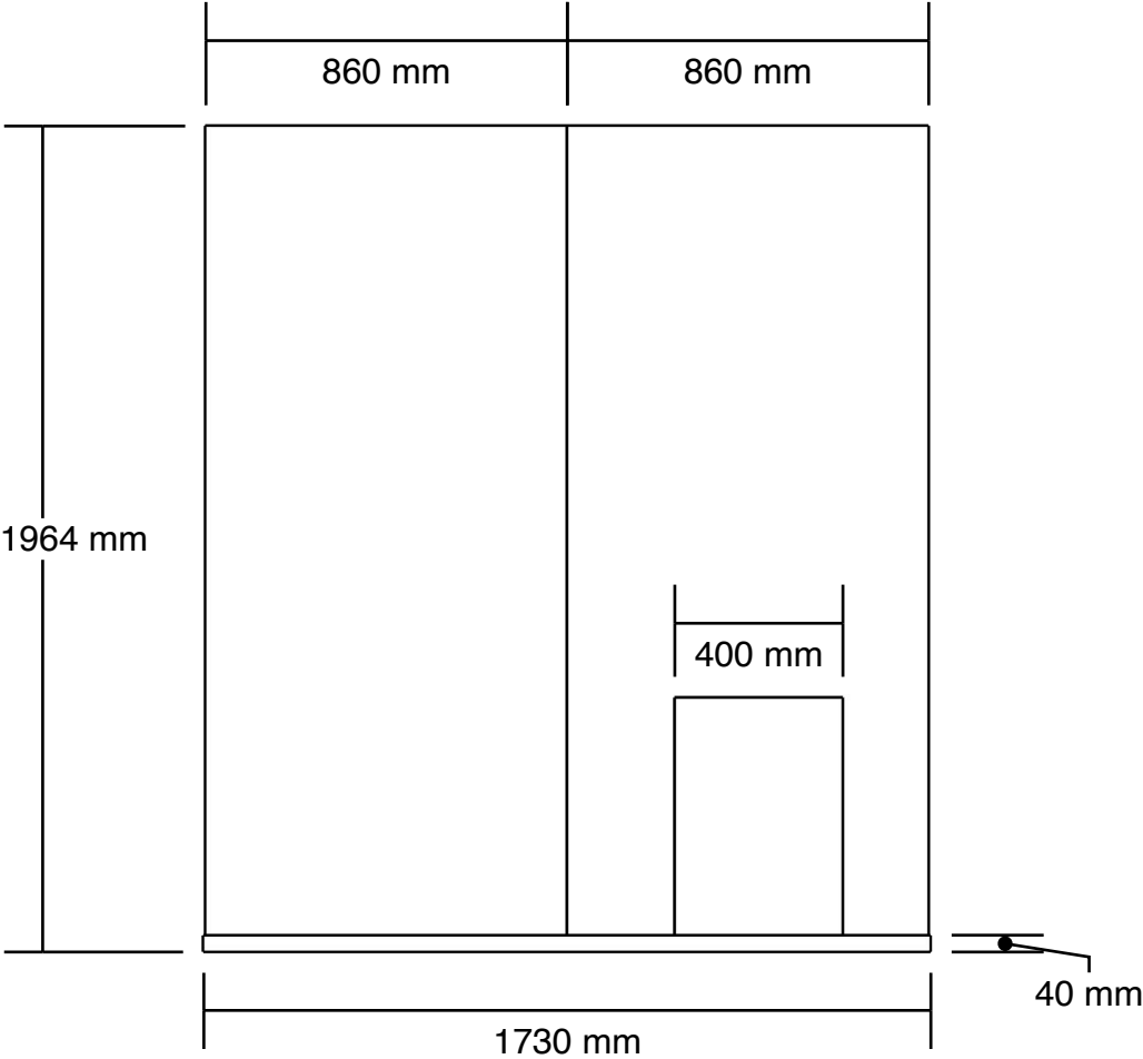
Elevation 1 1:20 @ A3
