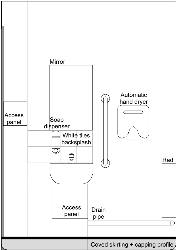
IE-03 01 Existing Dis. WC 1:20
