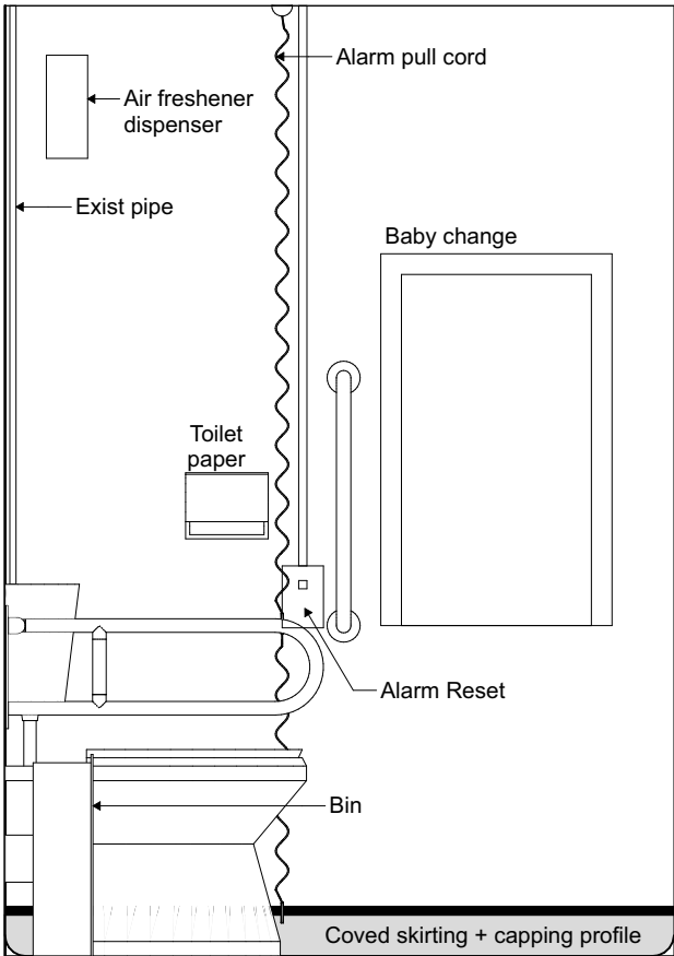
IE-03 03 Existing Dis. WC 1:20
