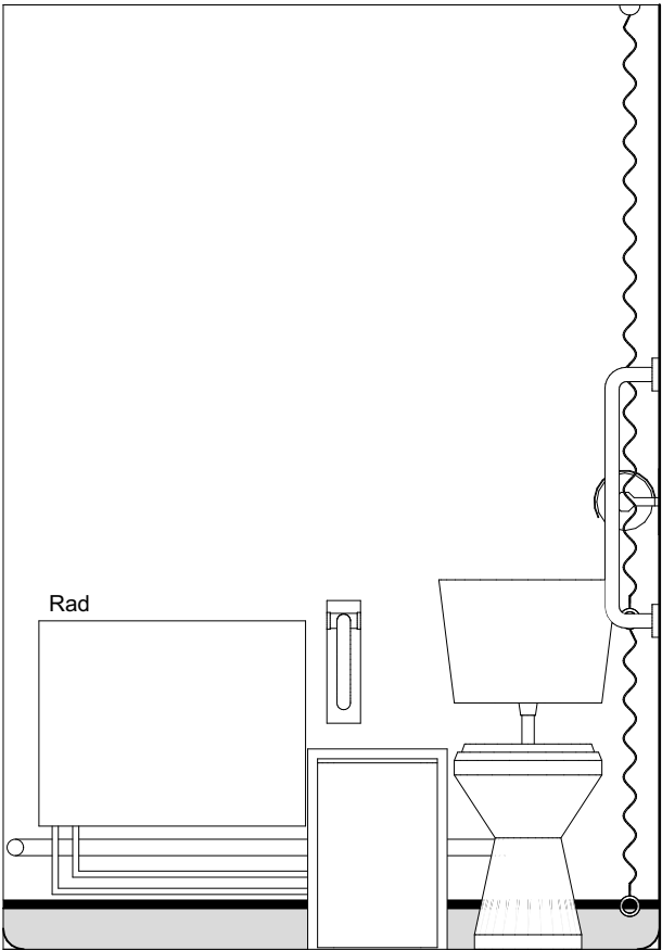
IE-03 02 Existing Dis. WC 1:20
