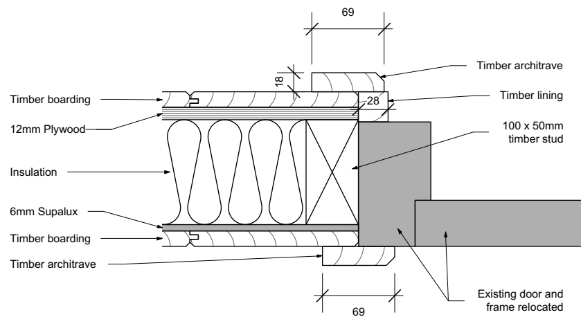
Door detail 1:5
