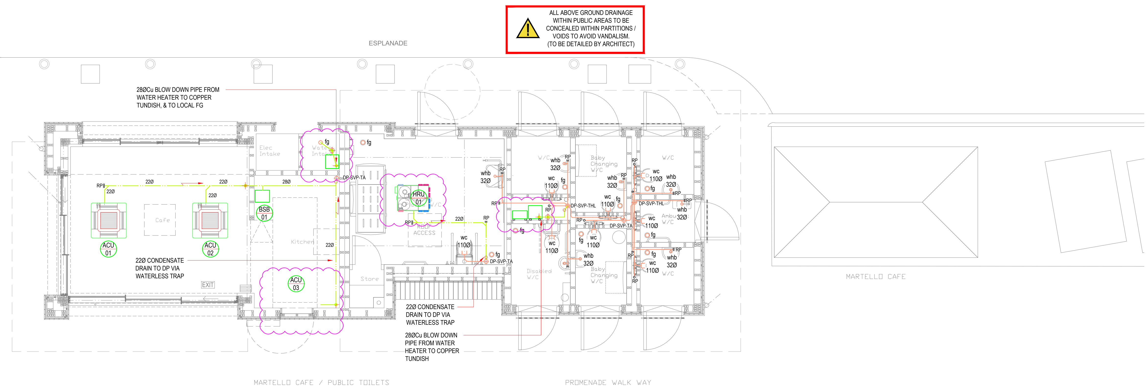
G r o u n d F l o o r P l a n
