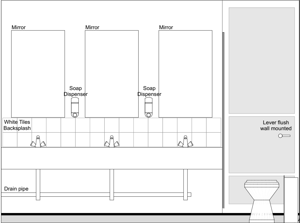
IE-02 03 Existing M-WC 1:20
