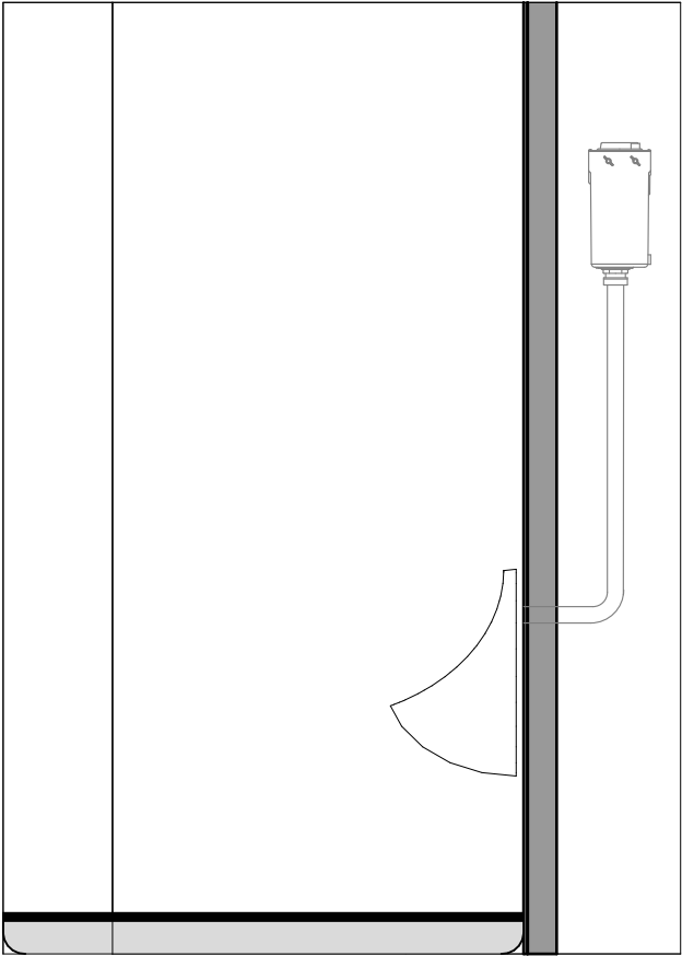
IE-02 07 Existing M-WC 1:20
