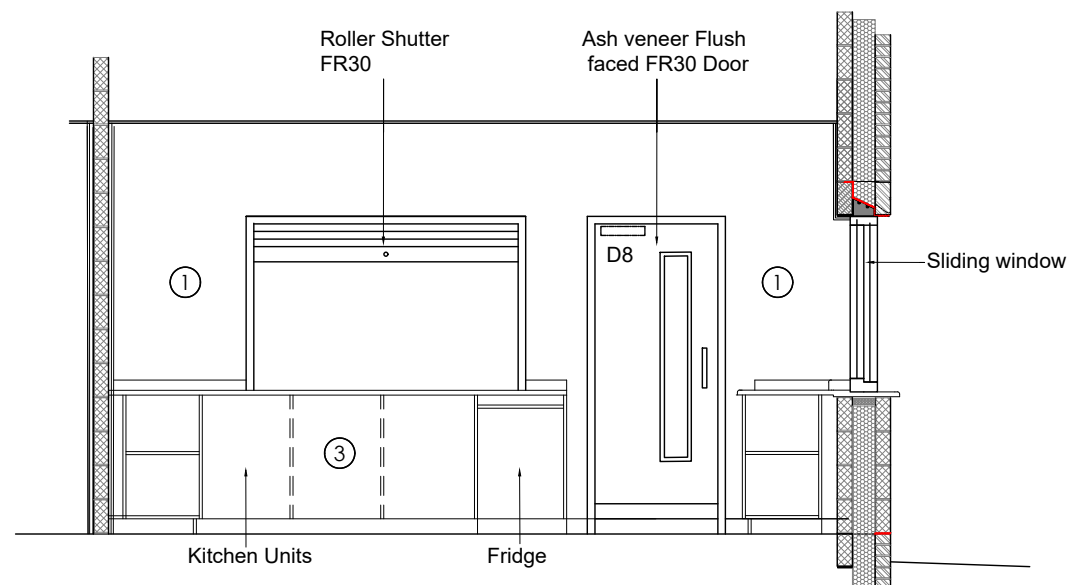
Elevation B
